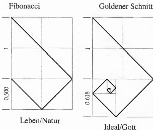
Abb. 8-10. Vergleich zwischen Fibonacci-Spirale und Spirale nach dem Goldenen Schnitt.
