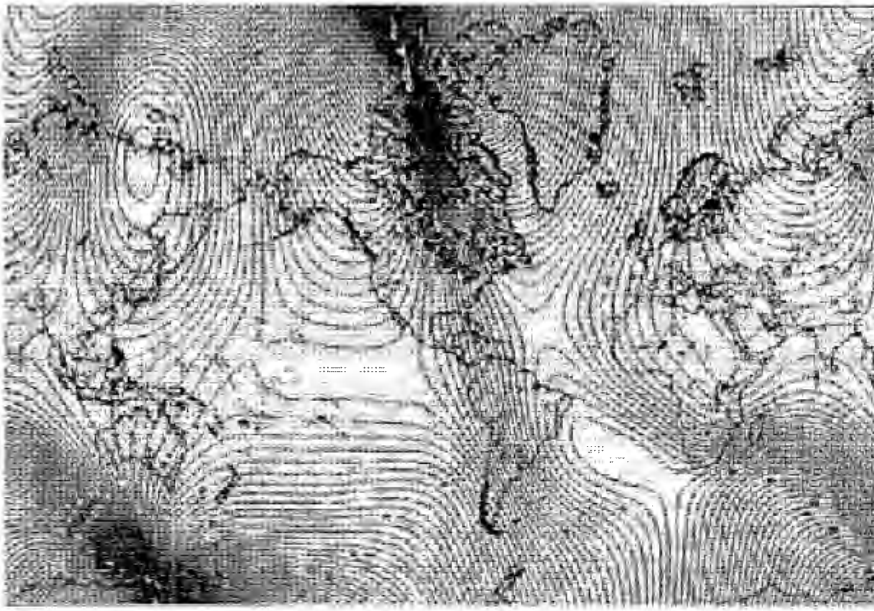
Abb. 2-44. Muster für ein komplexes Modell des wichtigsten Magnetfelds der Erde für das Jahr 1995, erstellt von einer US-Regierungsstelle.
