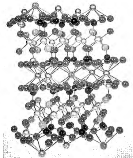
Abb. 6-33. Komplexe Molekülformation.
