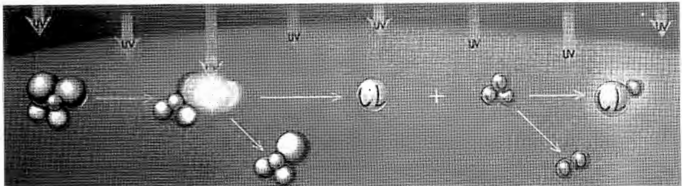
Abb. 3-5. Ozonreaktion bei Molekülen.
