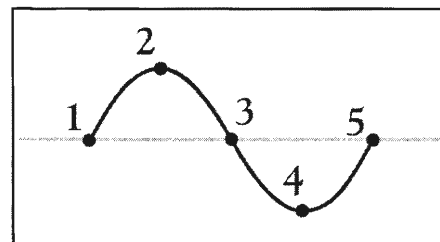
Abb. 8-13. Wellenform mit 5 Nullpunkten.
