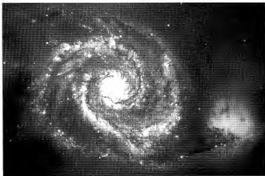
Abb. 8-30. Wirbelnde Galaxie.
