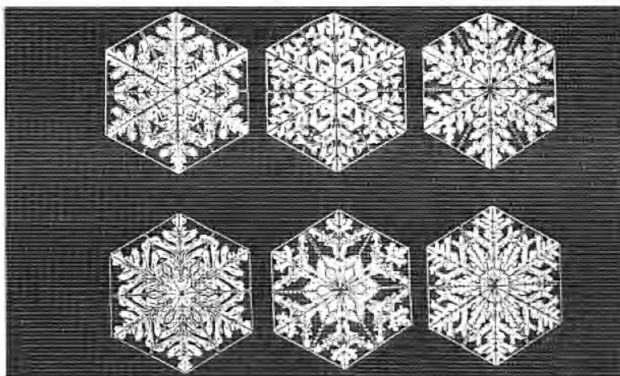
Abb. 6-46. Eiskristalle oder Schneeflocken.
