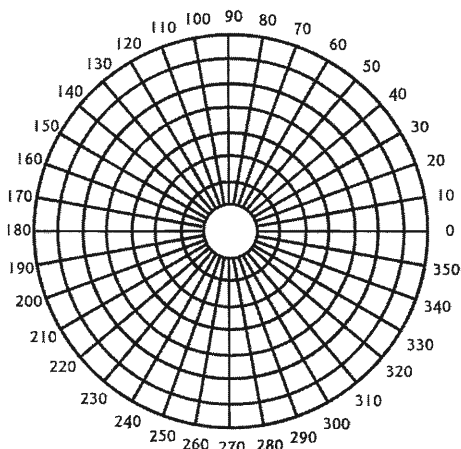
Abb. 8-22. Polardiagramm.
