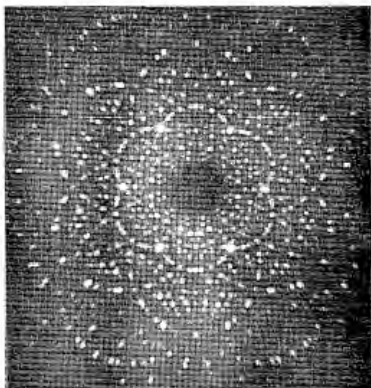
Abb. 6-28. Atomares Muster eines Beryllkristalls.
