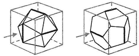
Abb. 6-48. Ikosaeder und Dodekaeder mit perfekter Einpassungsmöglichkeit in Würfel.
