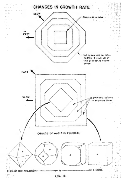
Abb. 6-36. Ein Fluoritkristall.
