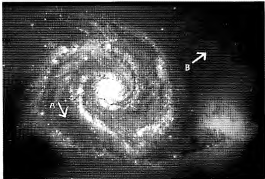
Abb. 2-35. Spiralgalaxie
