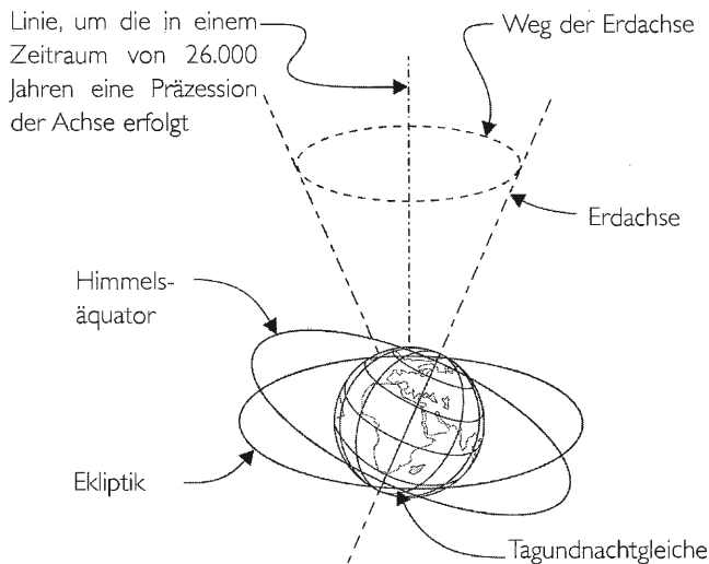
Abb. 2-39 Die Präzession der Tagundnachtgleichen (Punkt, an dem der Himmelsäquator der Erde ihre Ekliptik schneidet) geht auf die langsame Drehung der Erdachse um eine Senkrechte zur Ekliptik zurück.
