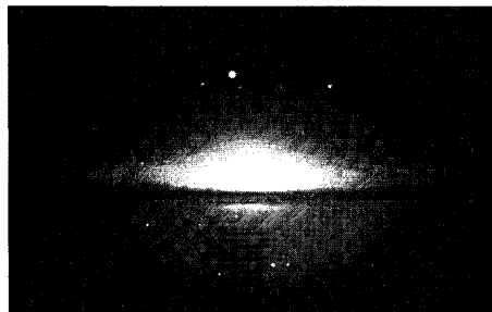
Abb. 2-38. Galaktische Hitzehülle.
