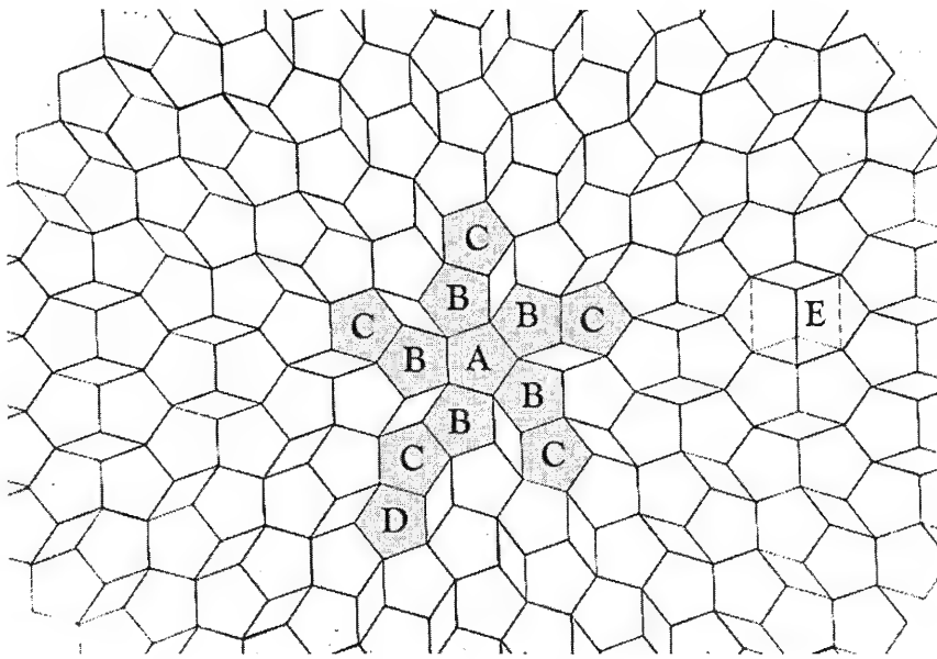
Abb. 6-23. Mackis aus Metatrons Würfel gewonnene Fünfeck-Konfiguration. Ausgeschnitten und gefaltet ergibt sich hieraus ein dreidimensionales Pentagonododekaeder (pentagonal dodecahedron).
