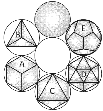
Abb. 6-15. Die fünf Platonischen Festkörper.
