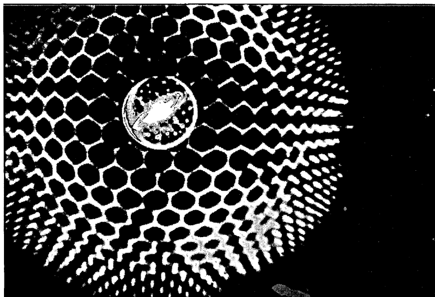
Abb. 2-37. Galaktische Energiekugeln.
