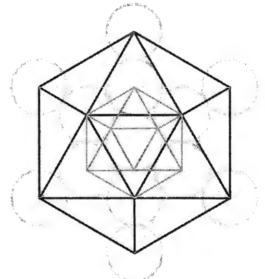
Abb. 6-19. Zwei aus Metatrons Würfel extrahierte Ikosaeder.
